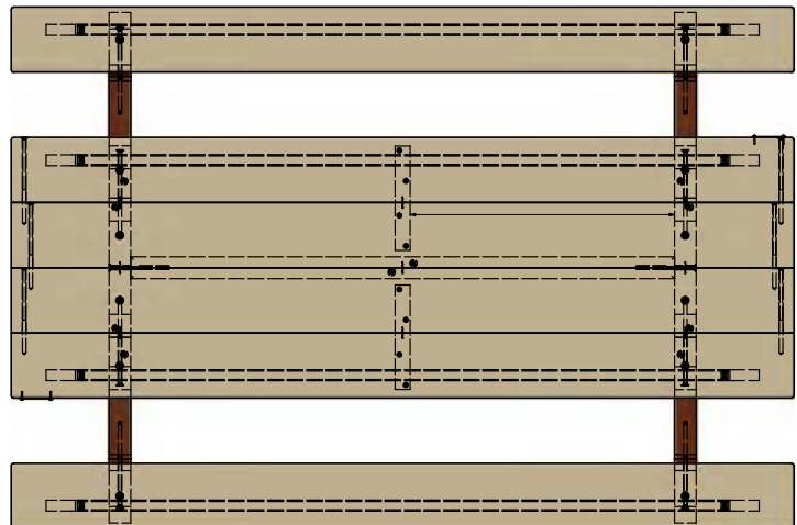
Metaalverstevingen in zowel het tafelblad als de zitvlakken.
